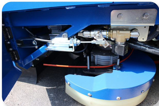
facile sostituzione e manutenzione delle spazzole
